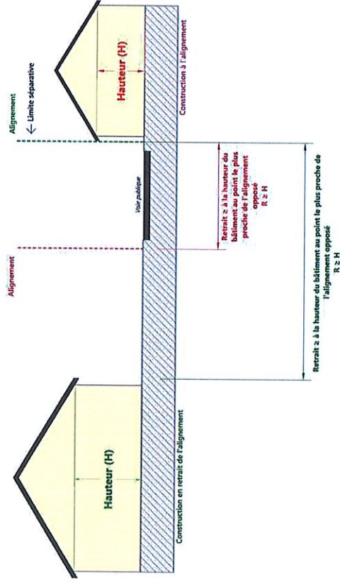
Schéma illustrant l'article R.111-16
